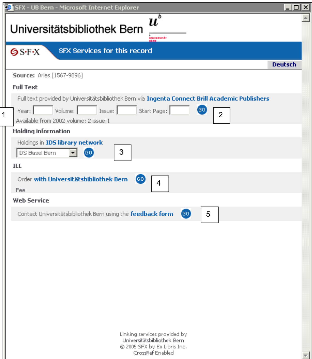
Abb. 3: SFX-Menu (Beispiel 1)
